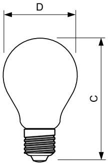
filament 7W-60W 806lm NAD 2700K E27D
